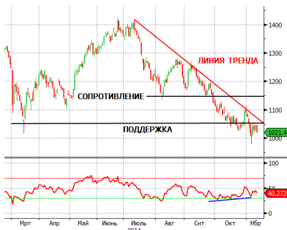
Рис.2 Индекс РТС
